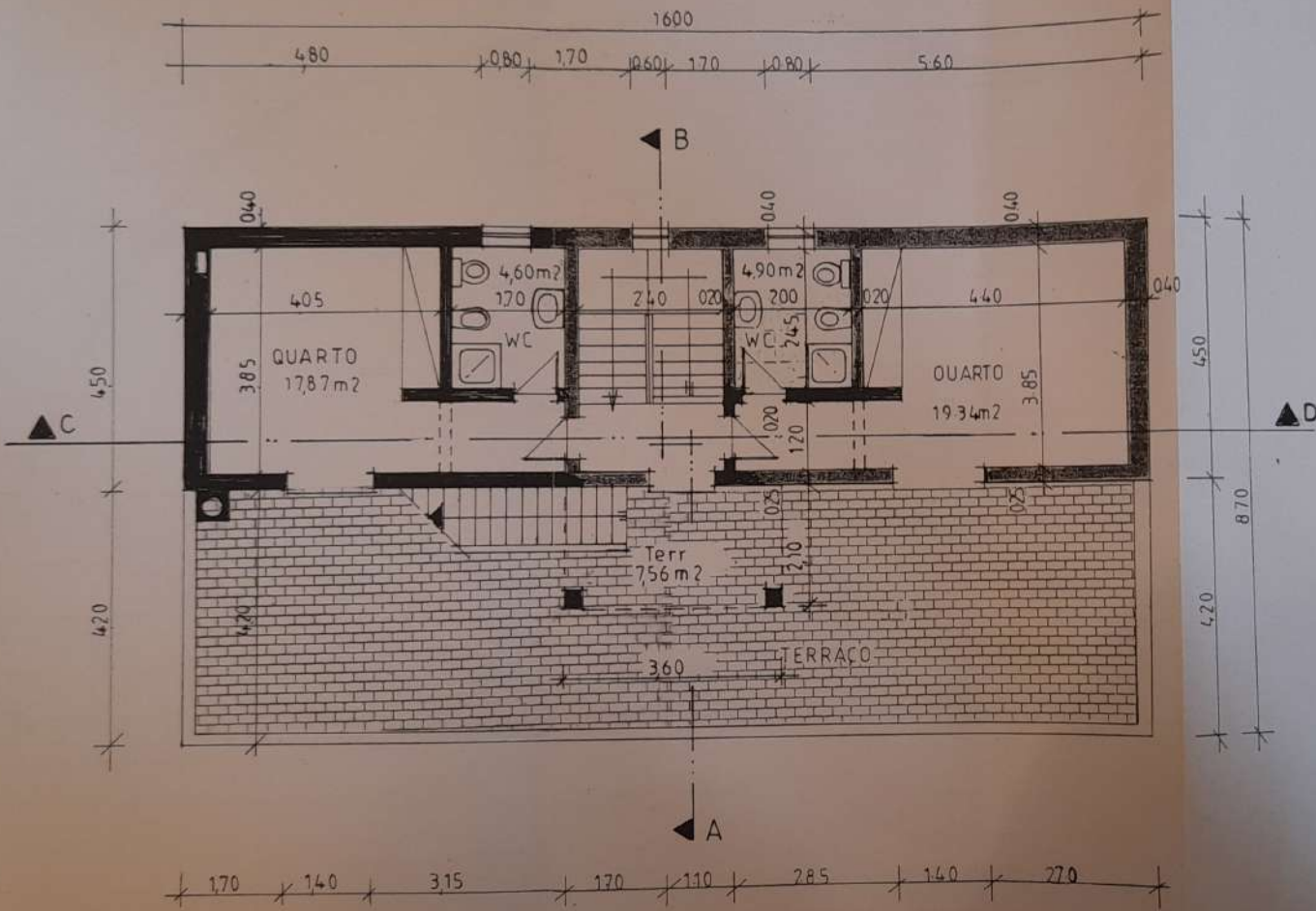
PLANTA DO 1º ANDAR
