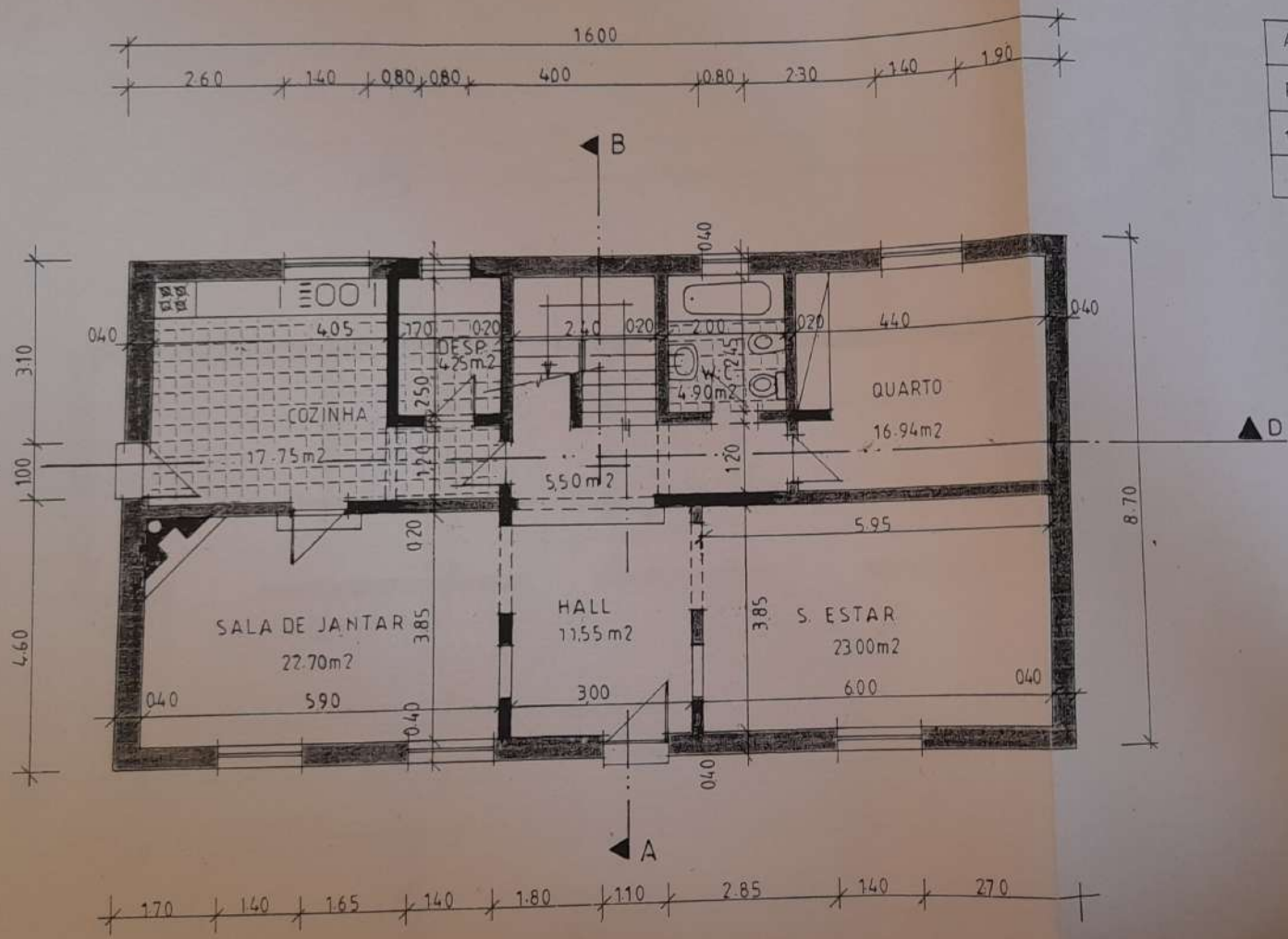
PLANTA DO R/CHÃO
